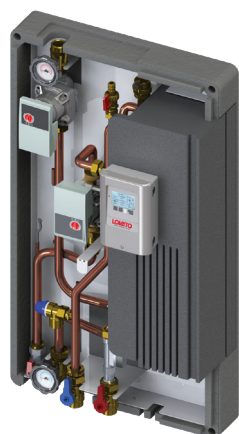
T-FAST ie40 Med elektroniskt reglerad blandningsventil på primärsidan. Kapacitet 40 l/min.
