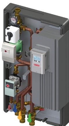
T-FAST ie60 Med elektroniskt reglerad blandningsventil på primärsidan. Kapacitet 110 l/min.
