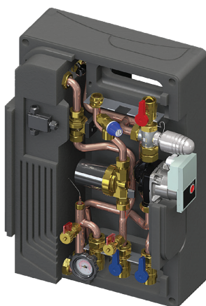
T-FAST i20 Med termisk blandningsventil på primärsidan. Kapacitet 30 l/min.
