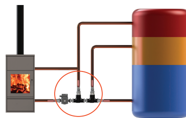
Laddomat 11-200 Duo Termiskt snabbbladdningskoppel
