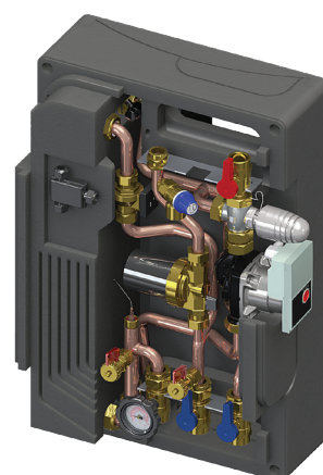
T-FAST i35 Med termisk blandningsventil på primärsidan. Kapacitet 34 l/min.
